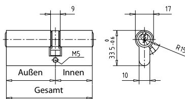
Sicherheits-Doppelzylinder mit 5 Stiftzuhaltungen
