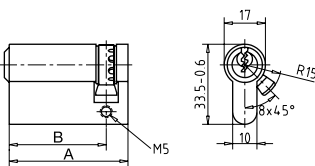
Sicherheits-Halbzylinder mit 5 Stiftzuhaltungen
